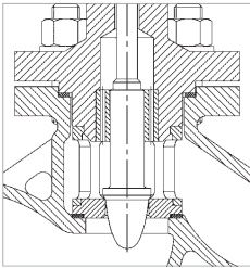
Клеточно-плунжерный затвор
