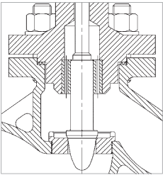
Плунжерный затвор
